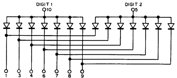
Fig. 14 TLM8051 (Display Unit D8)
